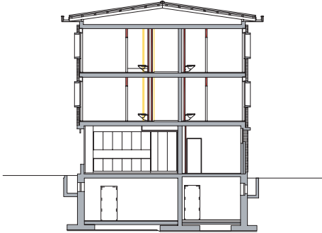
Querschnitt
