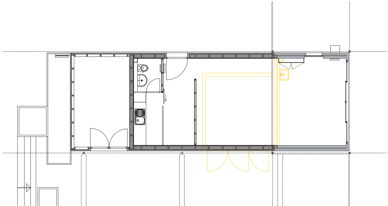
Grundriss
