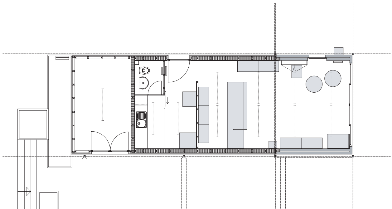
Grundriss Einrichtung
