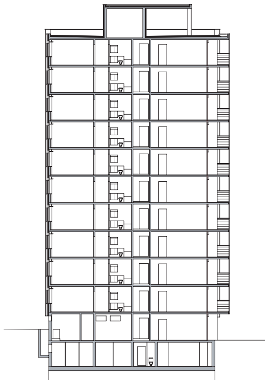
Schnitt
